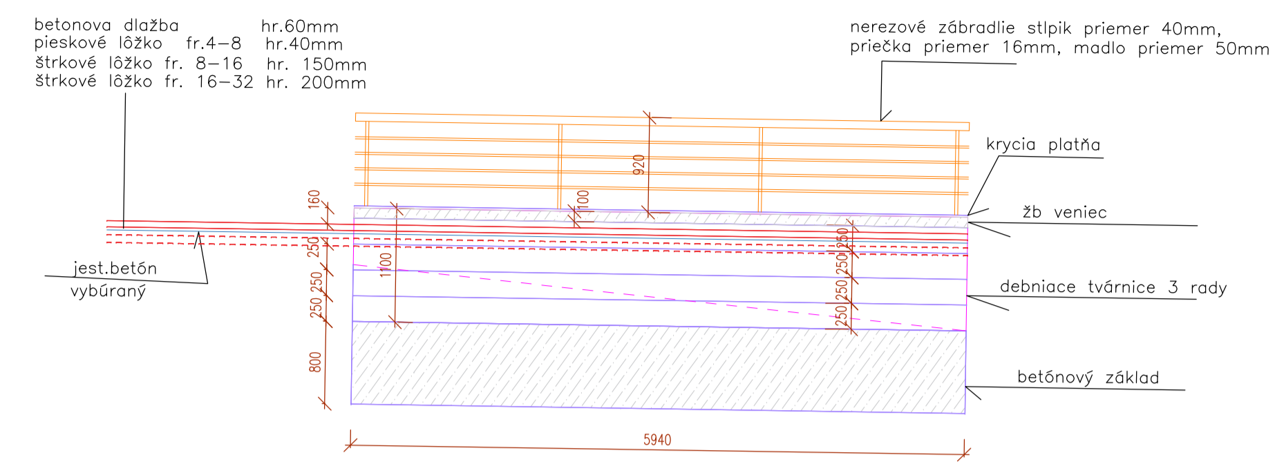
REZ A-A
